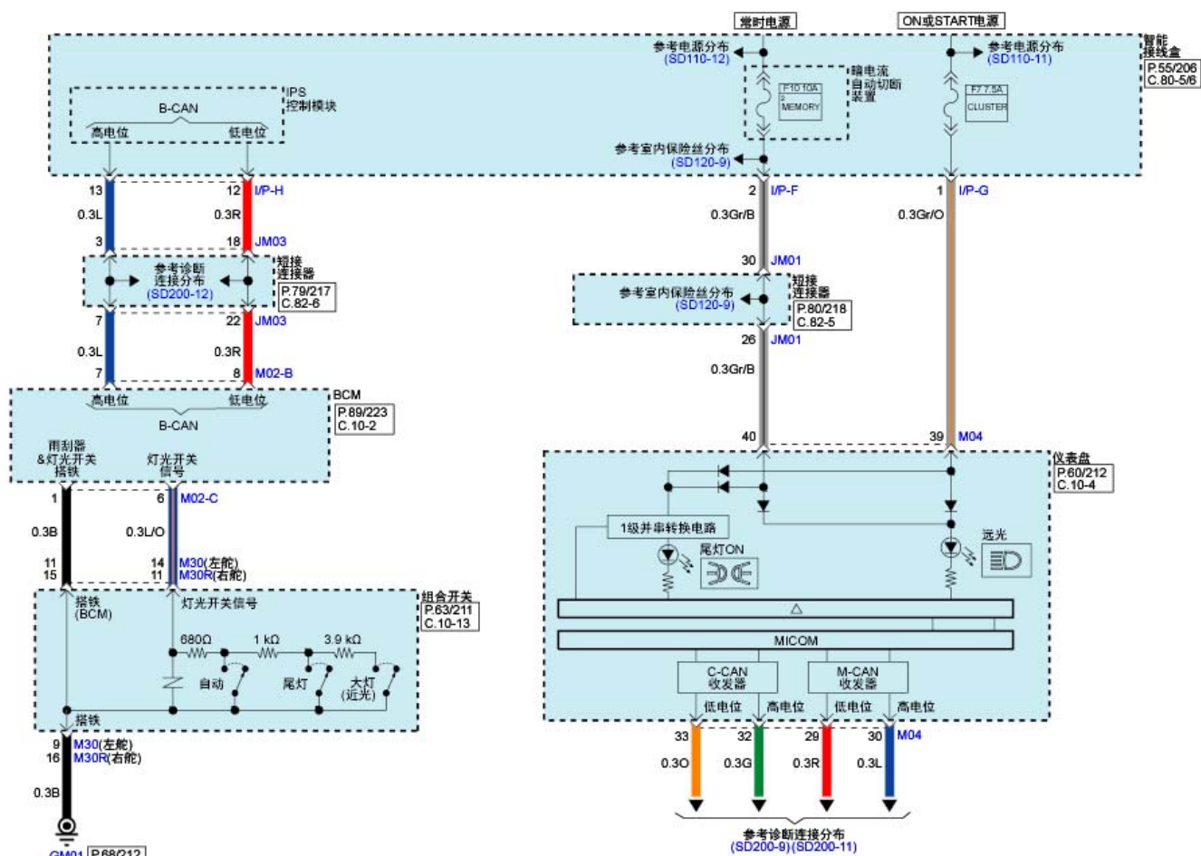
尾灯、驻车灯&amp;牌照灯(1)
